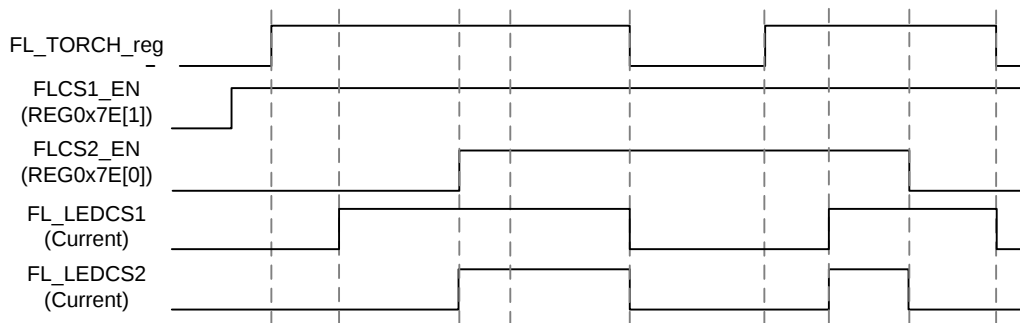
Figure 4-14. FLCS1_EN and FLCS2_EN (FL_TORCH_reg)
