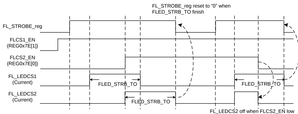
Figure 4-12. FLCS1_EN and FLCS2_EN (FL_STROBE_reg)
